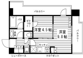
1LDKタイプ (36.9㎡)
